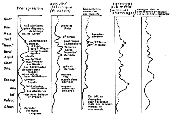
Mise en parallèle des principaux phénomènes observés dans le Sud-Est de l'Espagne depuis le Sénonien
