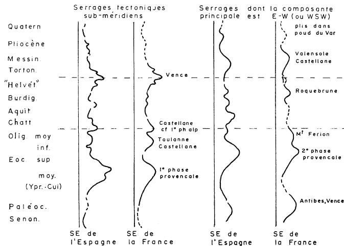
CHRONODIAGRAMMES TECTONQUES COMPARATIFS
